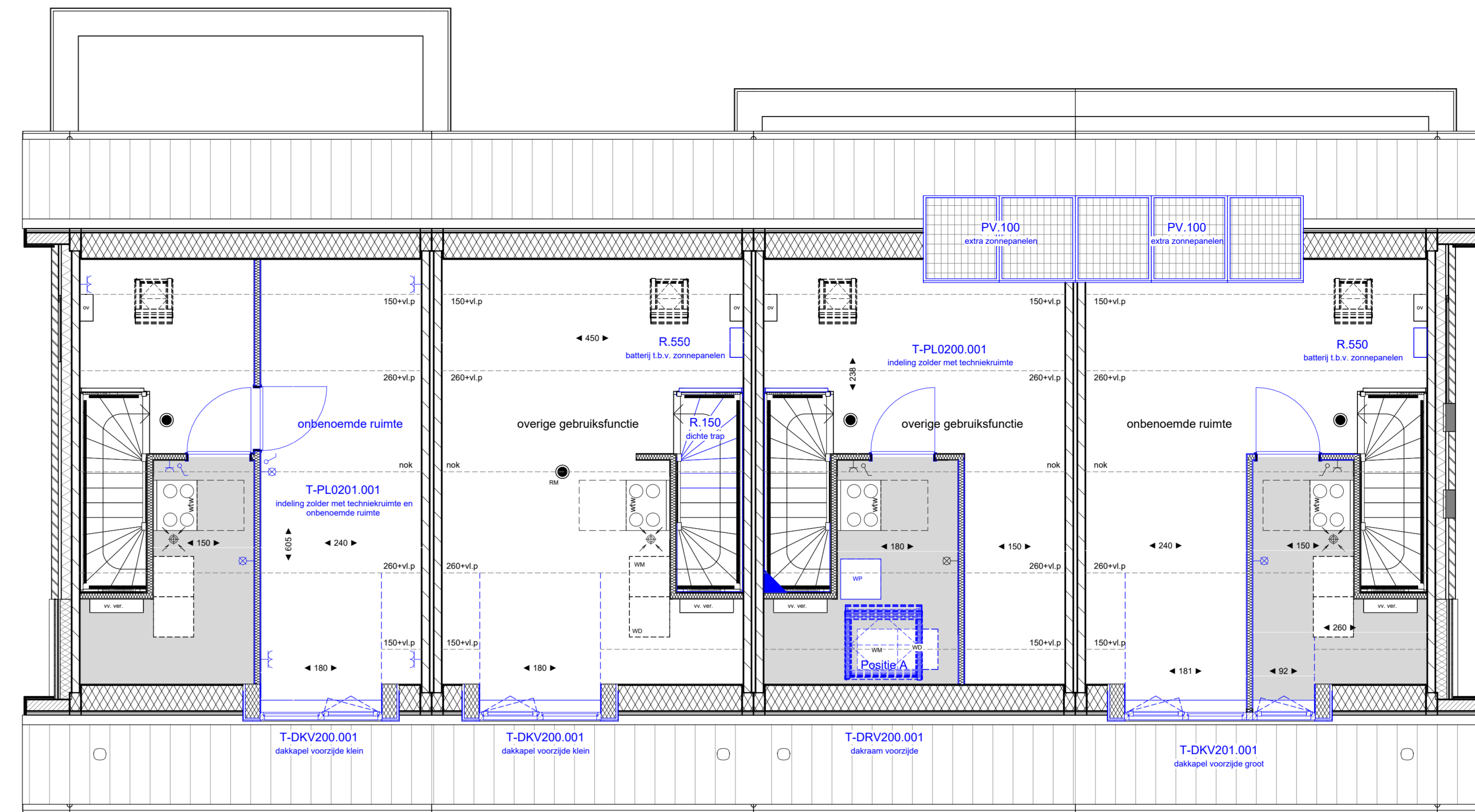
2e verdieping
