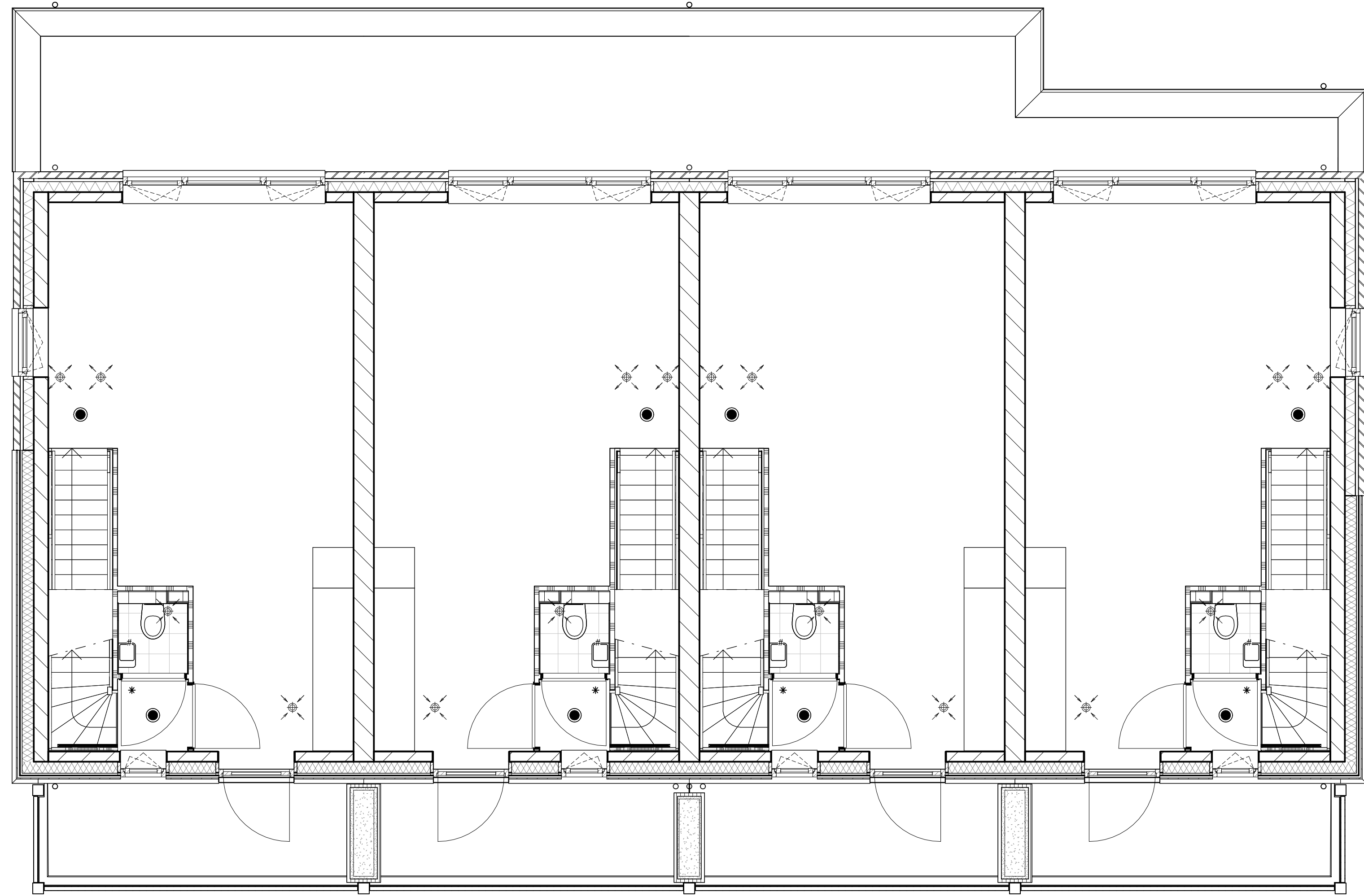
1e verdieping
