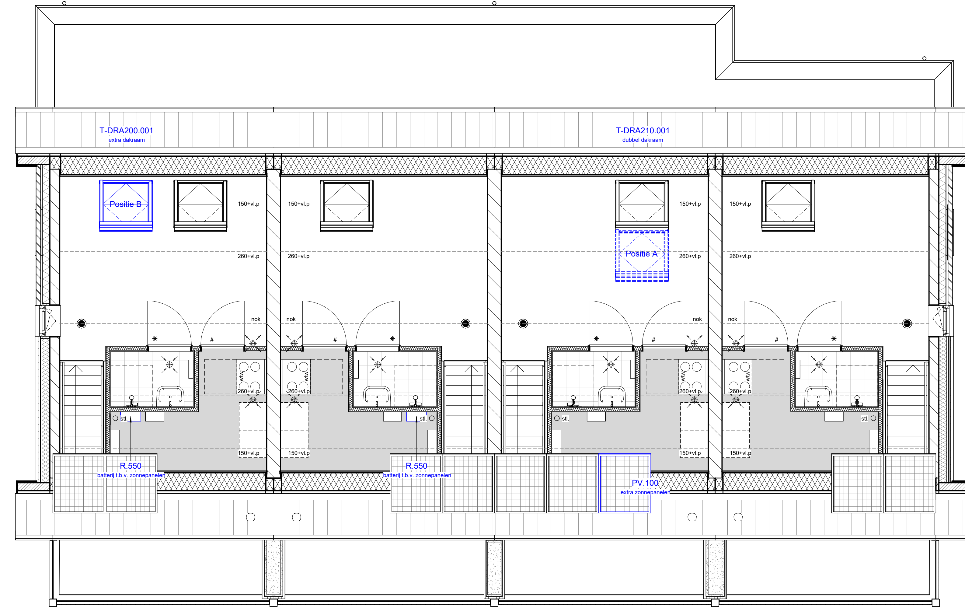
2e verdieping
