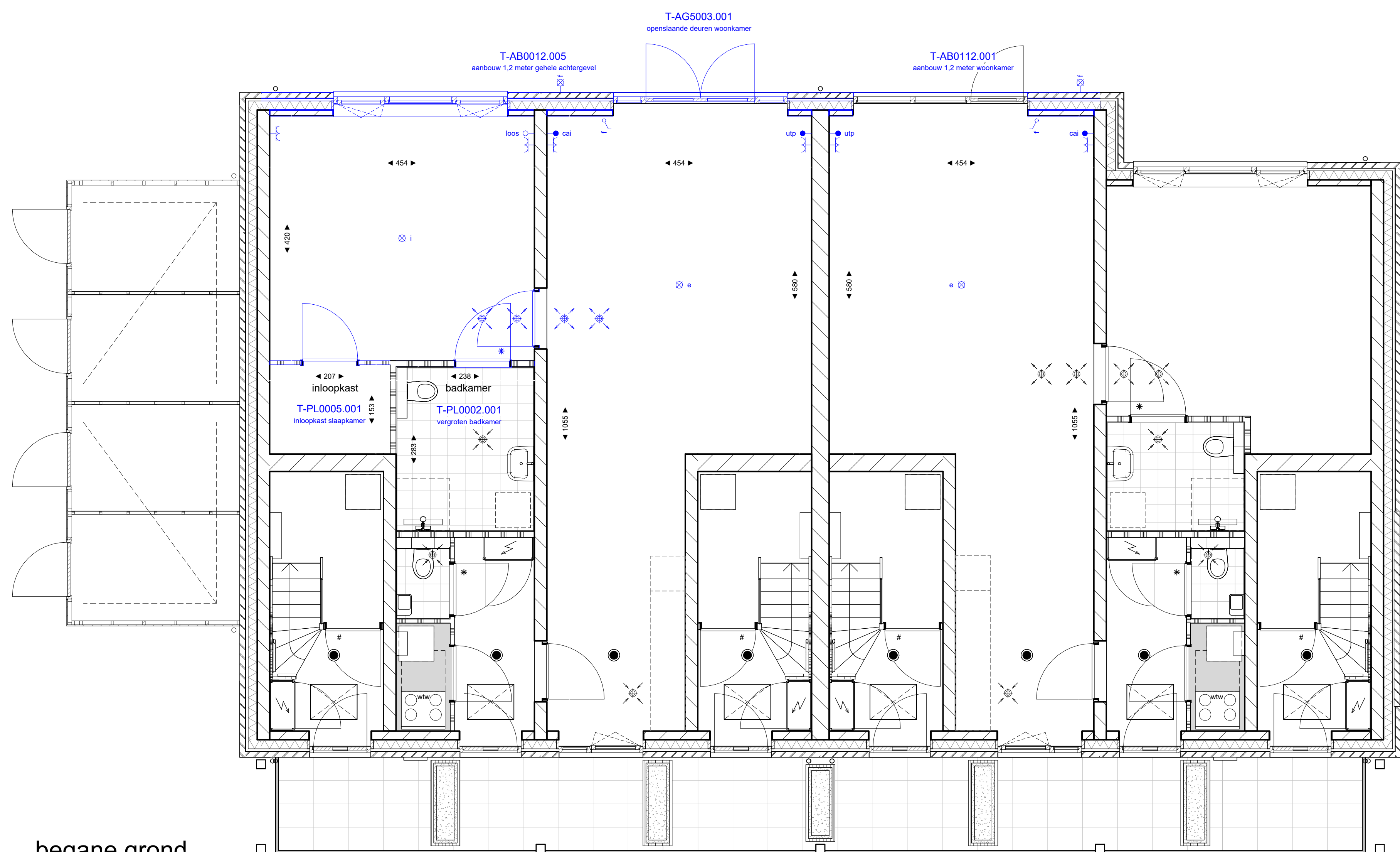
begane grond
