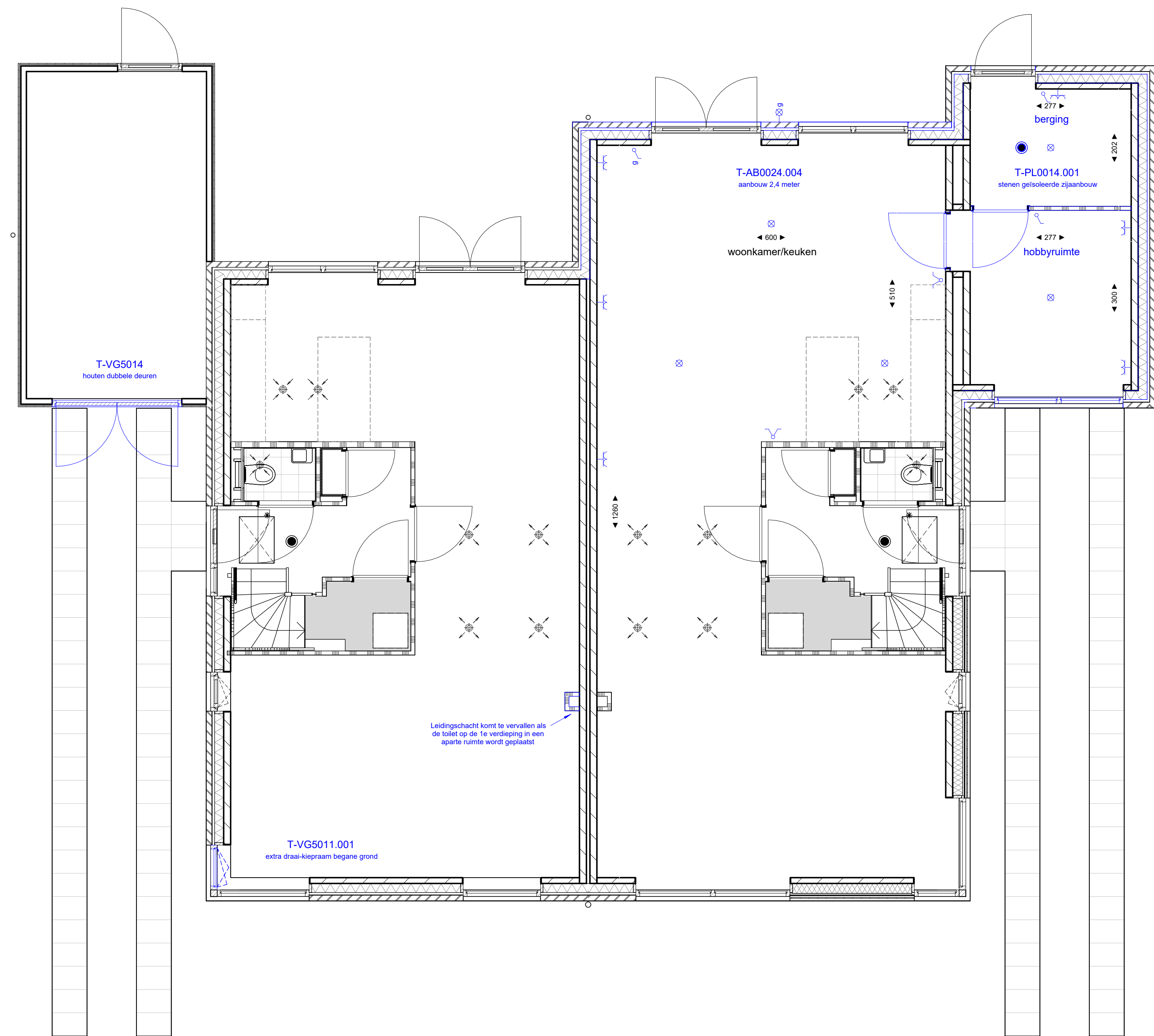
begane grond
