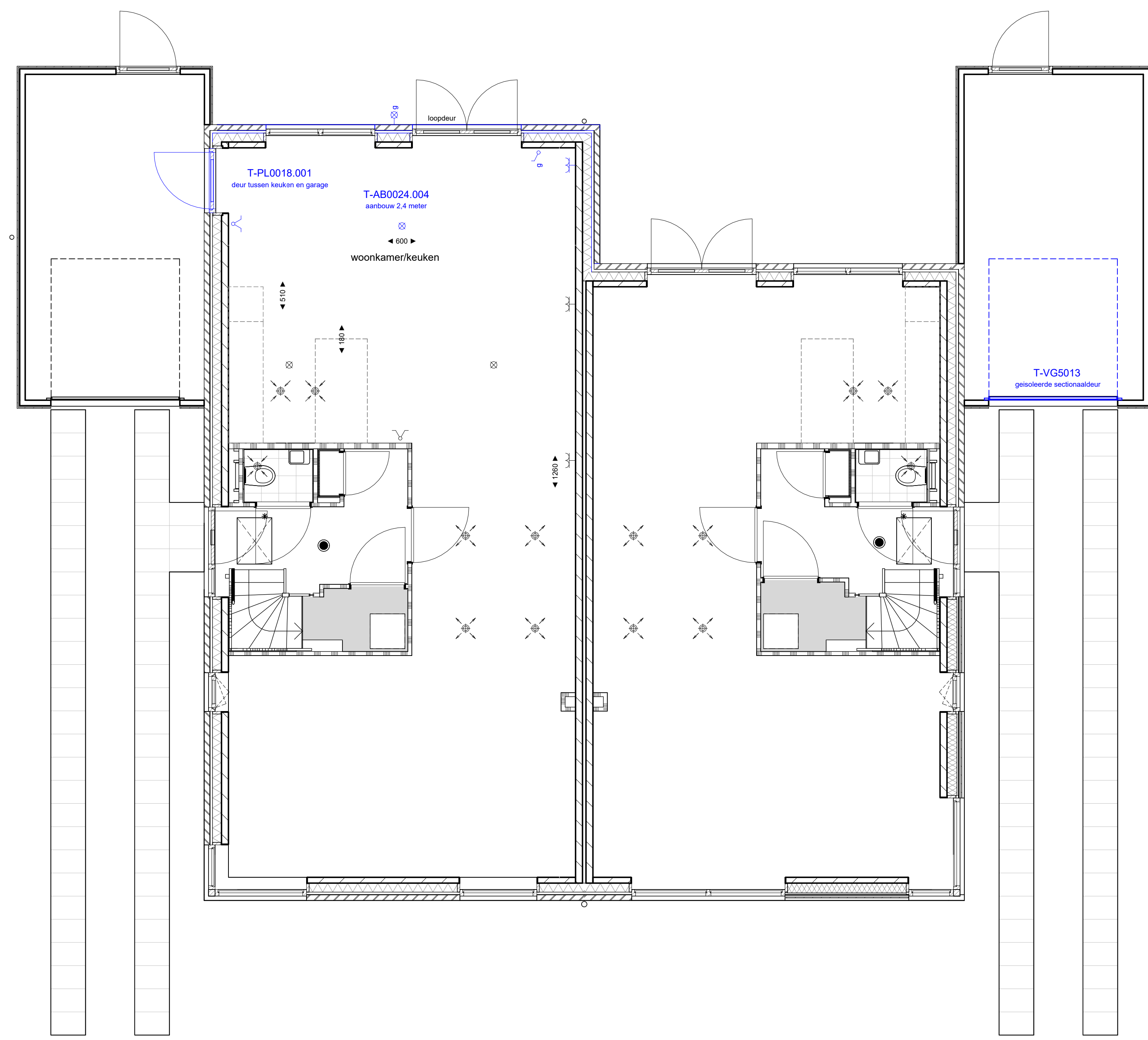
begane grond
