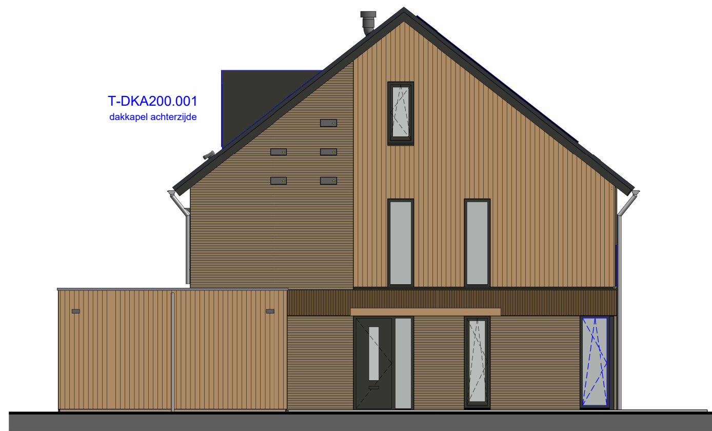
linkergevel
