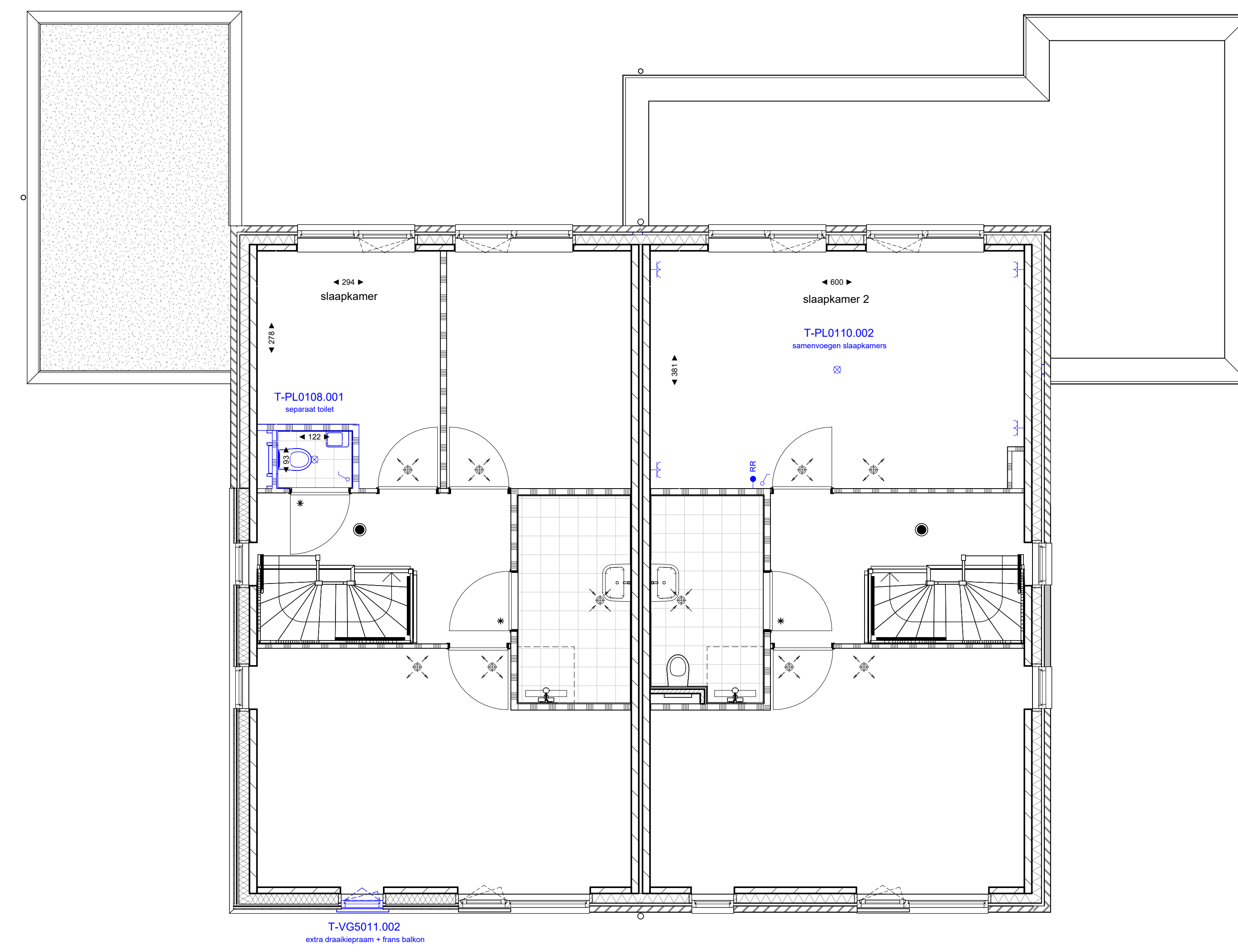
1e verdieping
