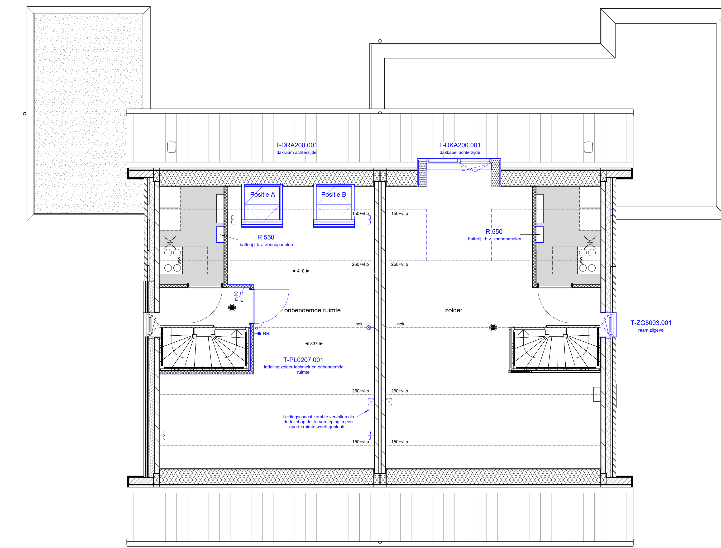
2e verdieping
